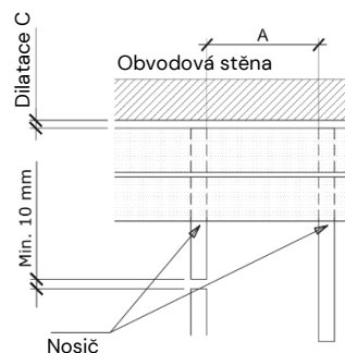
Obr. 2 Pokládka nosičů a vzdálenost mezi nimi
