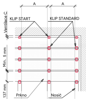
Obr. 4 Minimální spáry mezi prkny a mezi prkny a pevnou zdi
